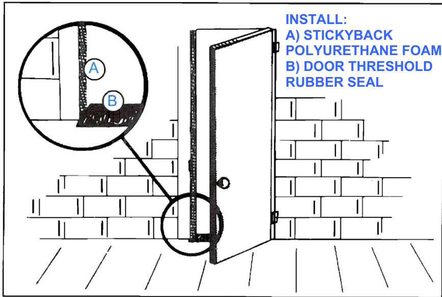
Fig. 12 DOOR SEAL
